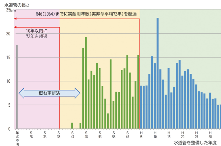
建設年度別の水道管の延長
