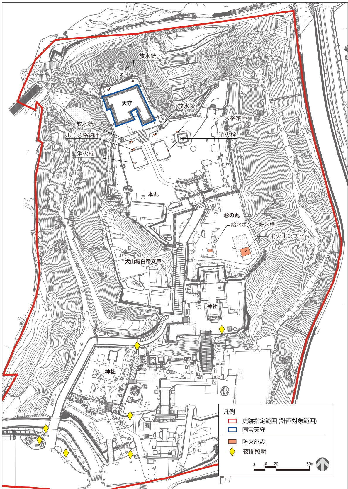
図 4.3 防火施設及び防犯設備の配置状況
