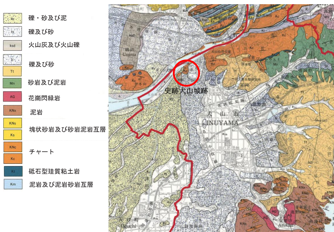
図 2.1 計画対象範囲周辺地質図（赤線は市境界）（地質調査総合センター 地質図表示システム 地質図 Navi、「5 万分の 1 地質図 岐阜」より抜粋、一部加工）
