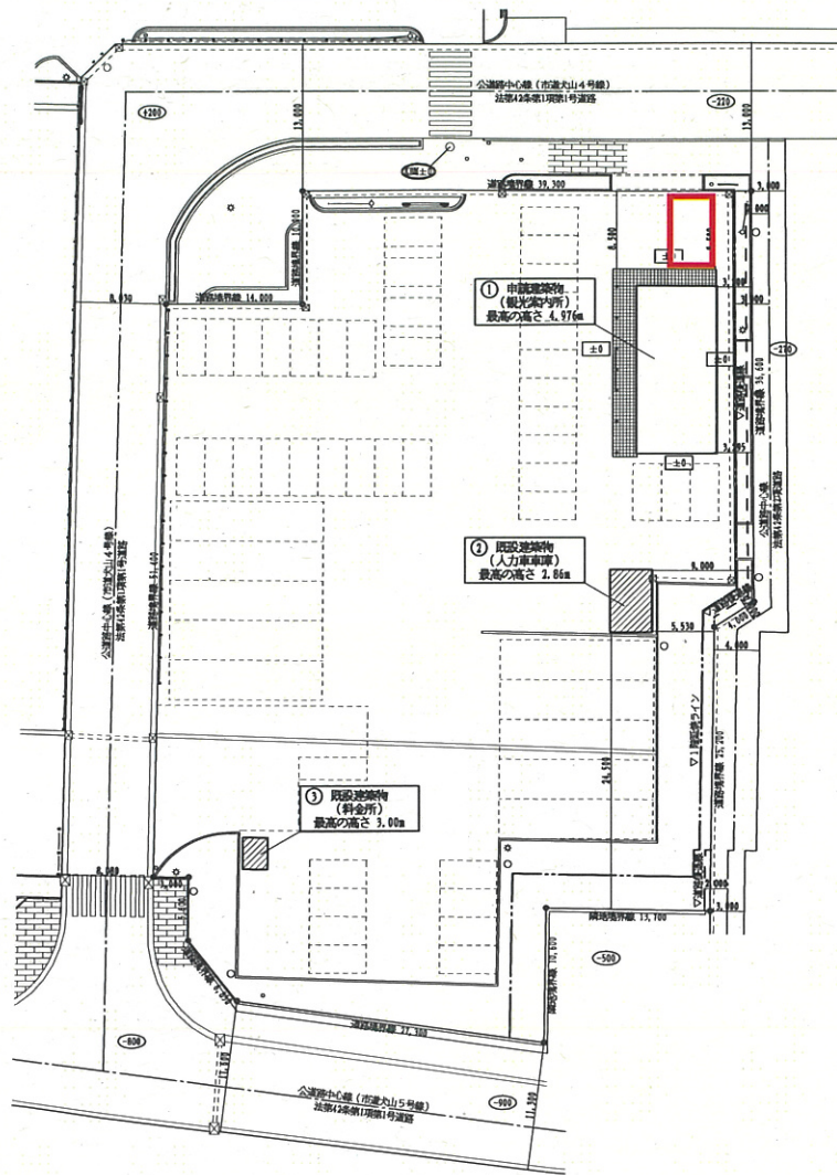
配置図 S=1/500 設計GL=KBM±0とする。(レベルは外欄図参照)
