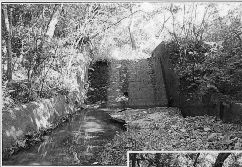
H29. 8. 18豪雨により落差工崩壊
