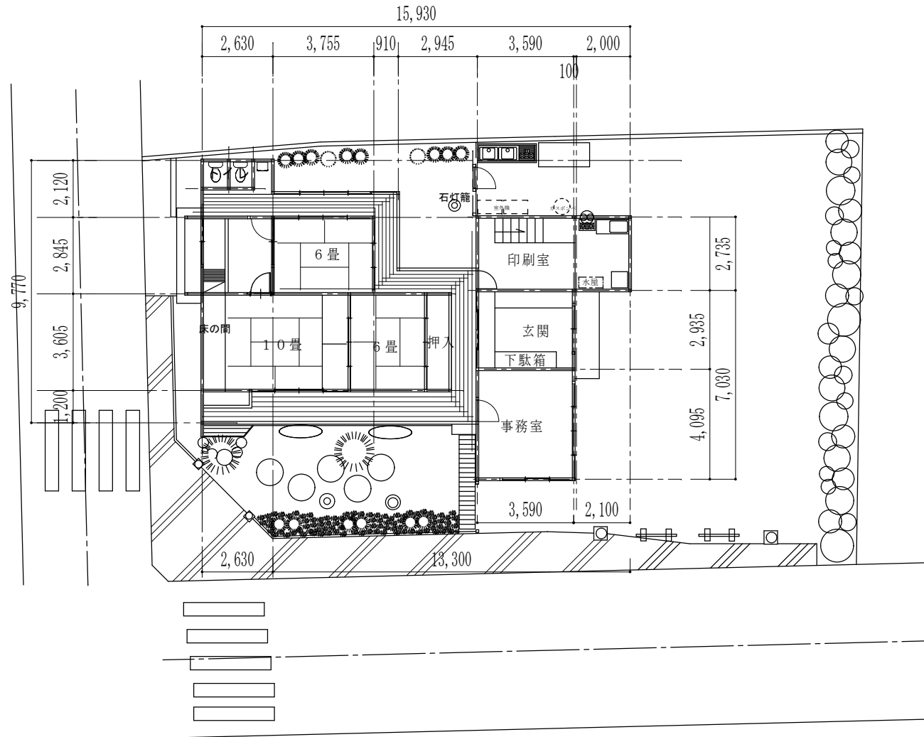
2階平面図
