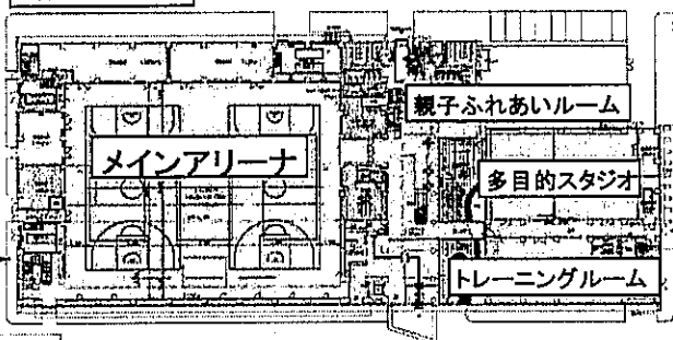
1階平面図
