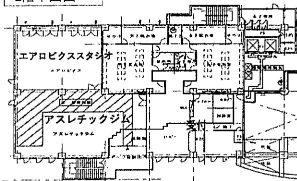
2階平面図
