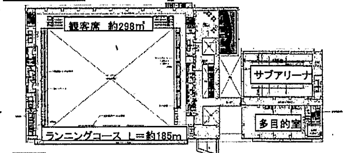
2階平面図
