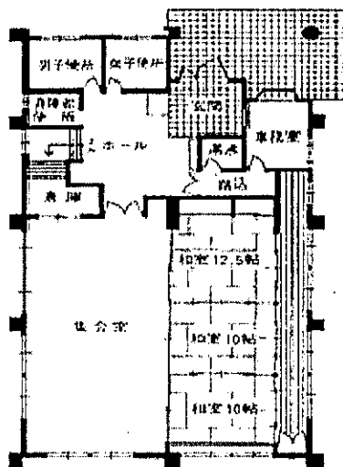
1階平面図
