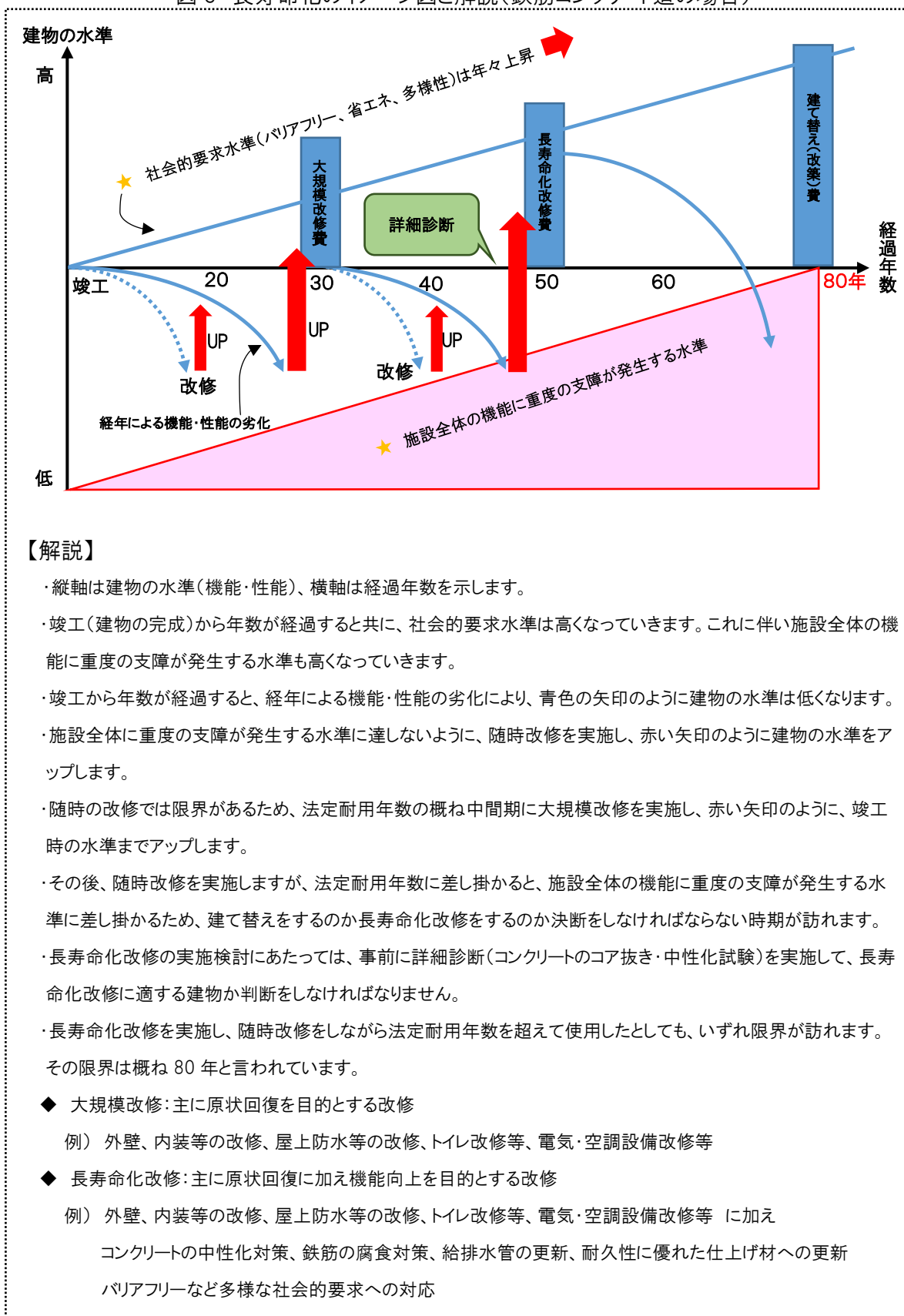
図3 長寿命化のイメージ図と解説(鉄筋コンクリート造の場合)
