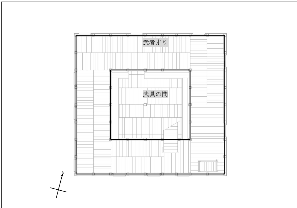
二階平面図
