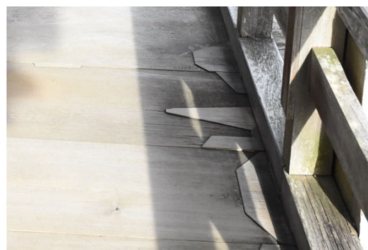
図 4.45 埋木による廻縁床板修理
