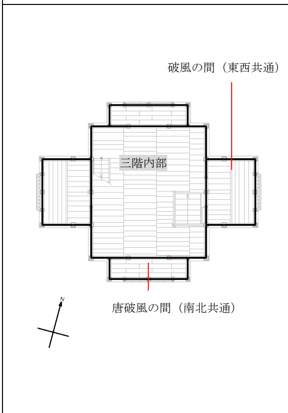
三階平面図
