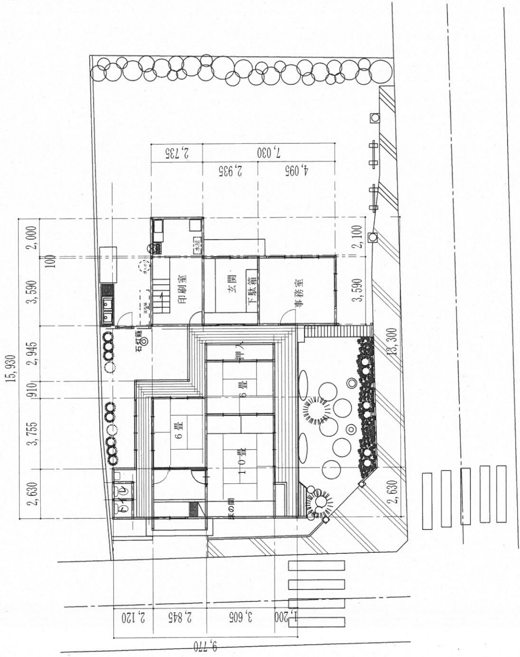
2階平面図
