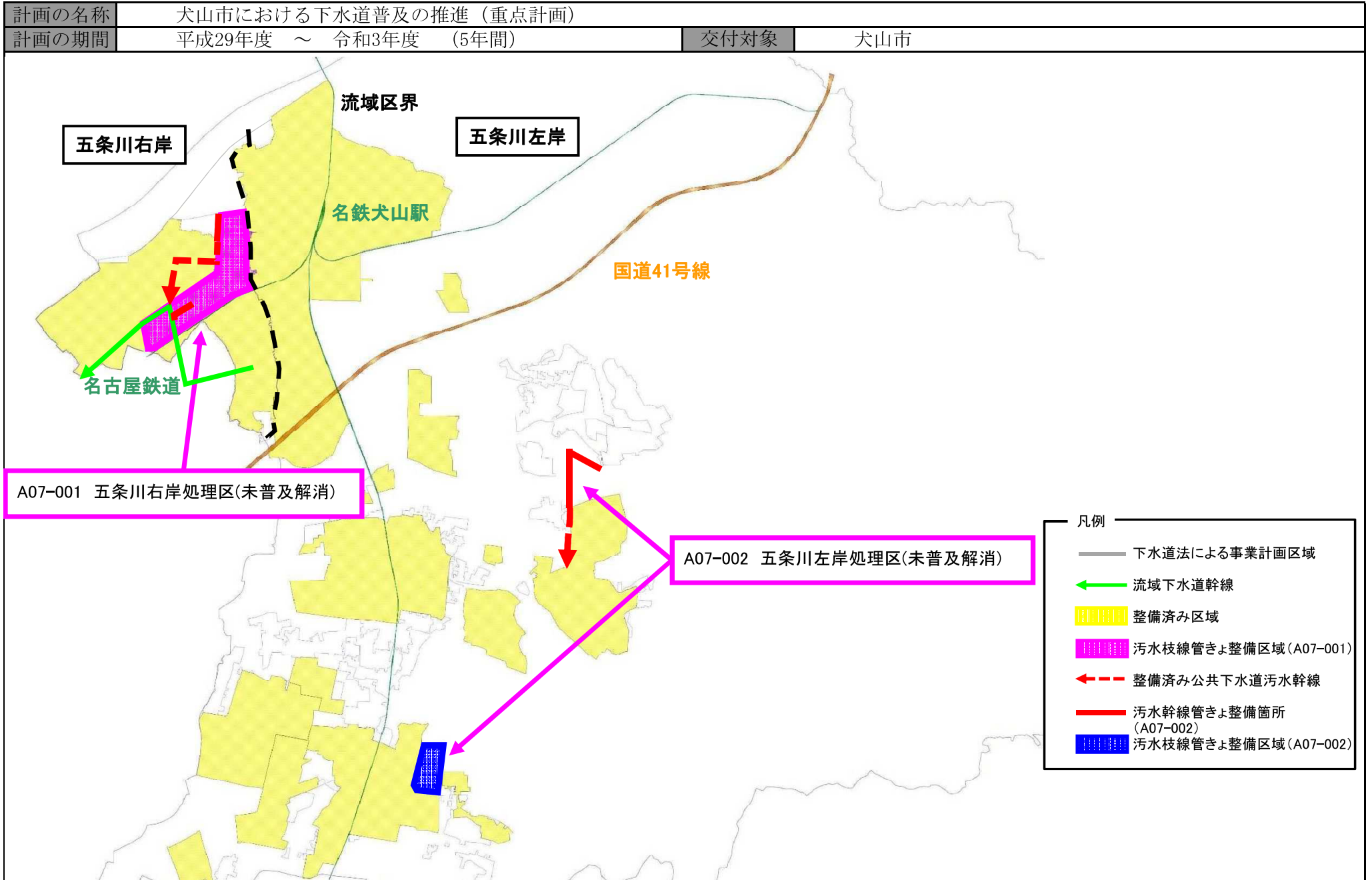
様式3 (参考図面)
