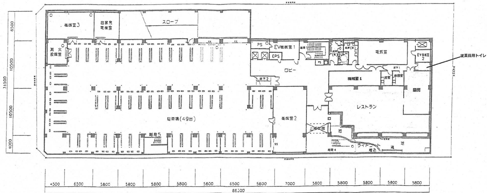
地下1階平面図(1/300)
