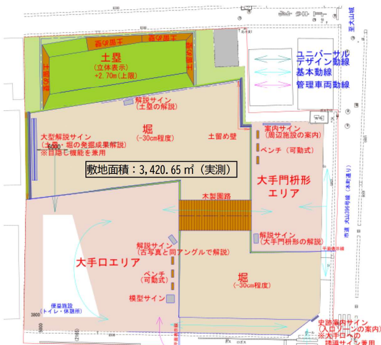
大手門枡形跡（犬山市福祉会館跡地）整備計画図 ※検討中
