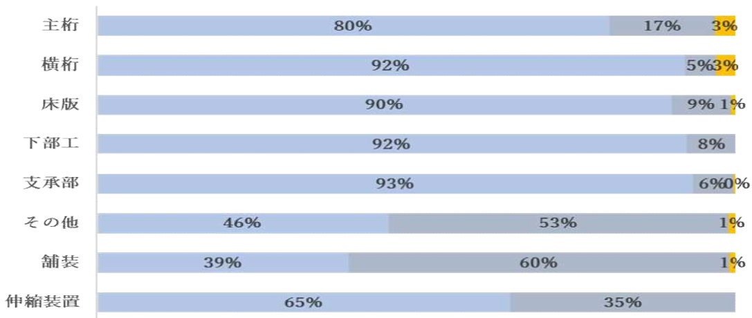
図-4.2 部材ごとの健全度評価
