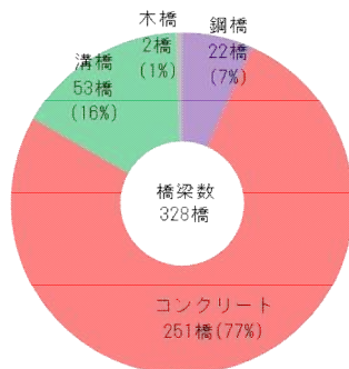
図-1.3 橋種別の橋梁割合
