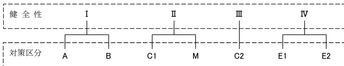
図-1.7 健全性に対策区分の関係性
