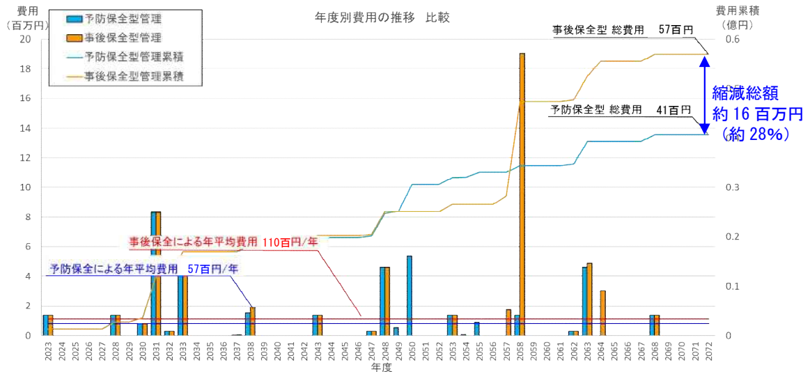
図-5.4 長寿命化修繕計画によるコスト縮減効果(歩道橋)
