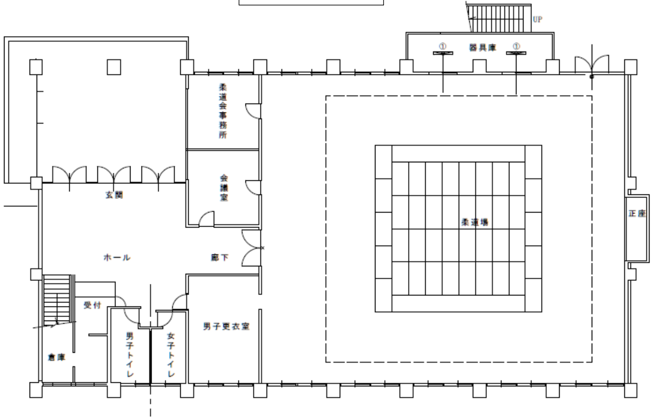
1階平面図
