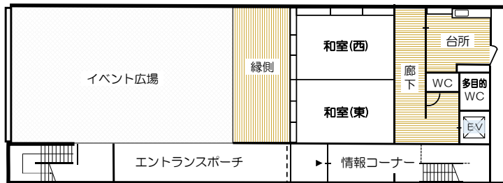
1階 平面図
