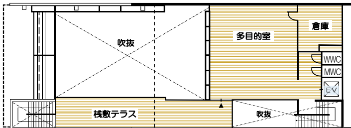
2階 平面図
