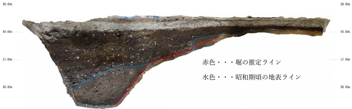
堀断面オルソ画像（東から）
