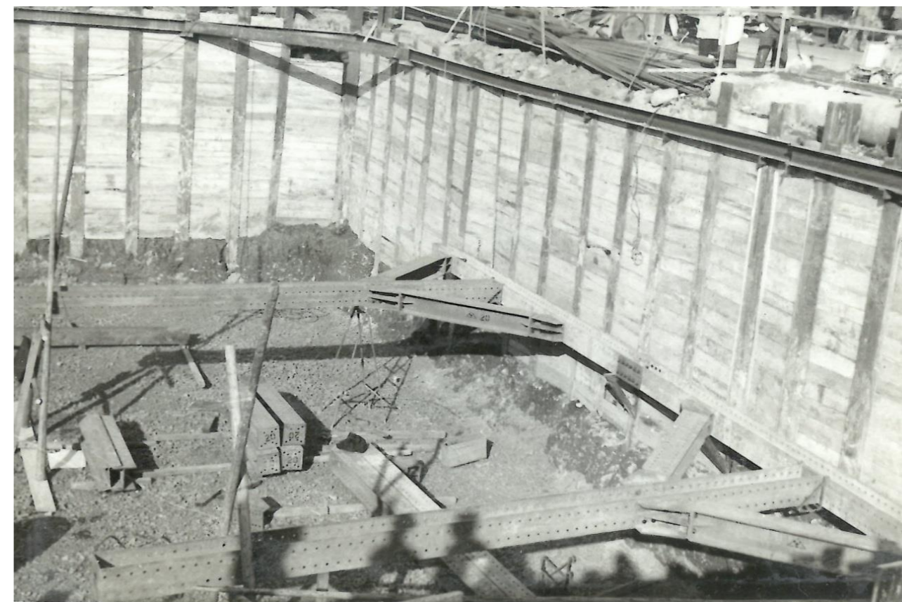
矢板設置完了（南西又は北西から）
